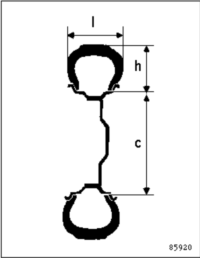
Exprimée en millimètres (ou en pouces) et mesurée à l'endroit le plus large du pneumatique l = 175 mm
